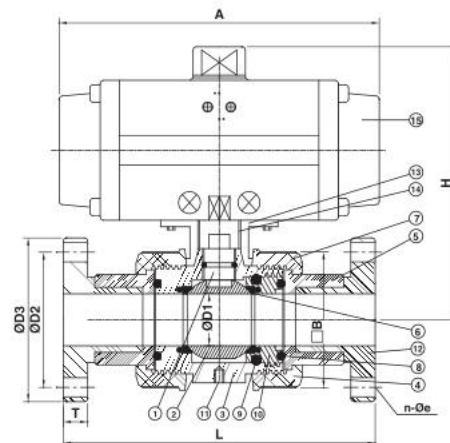
DN65~DN100 FLANGE TYPE
